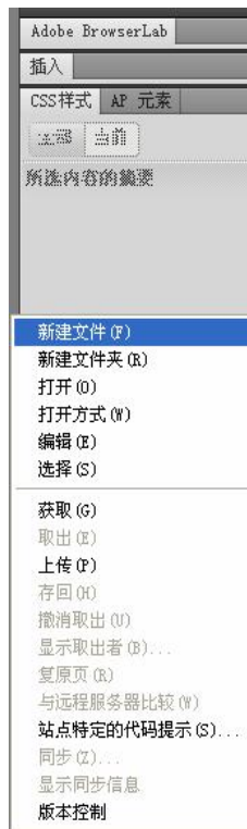
图 2-15 创建文件
