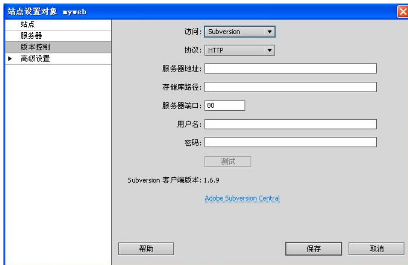
图 2-6 版本控制
